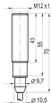
Габаритный чертеж
